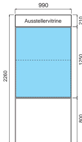
Frontansicht
